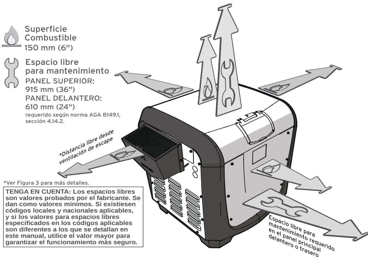
Figura 2. Espacios libres
