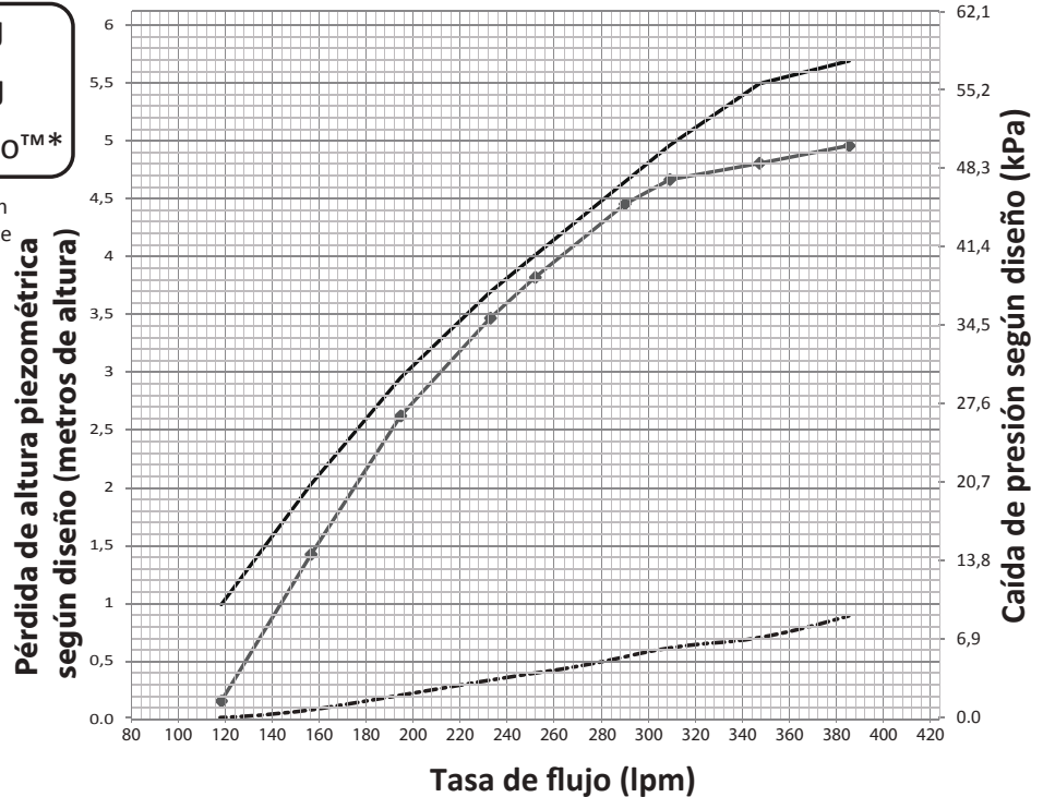
Figura 7. Gráfico de pérdida de altura piezométrica
