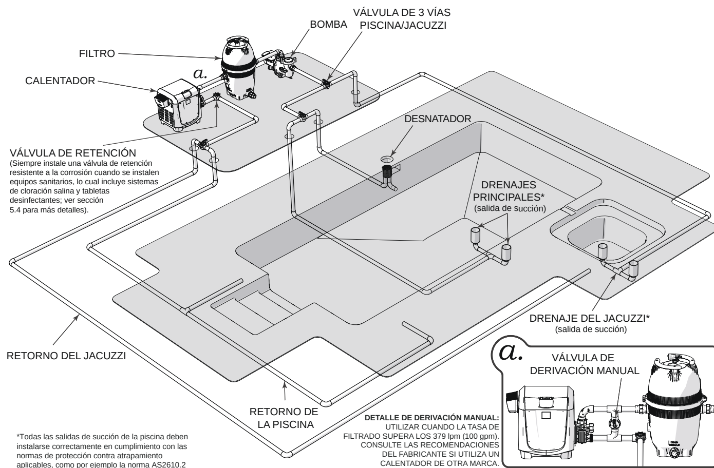
Figura 6. Configuración típica de la cañería de agua
