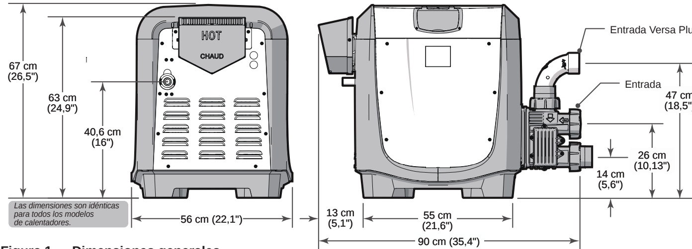
Figura 1. Dimensiones generales
