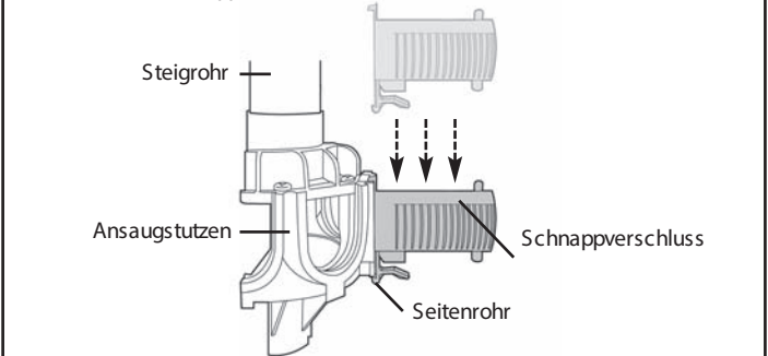
ABBILDUNG 1 - Schnappverschluss-Detail
