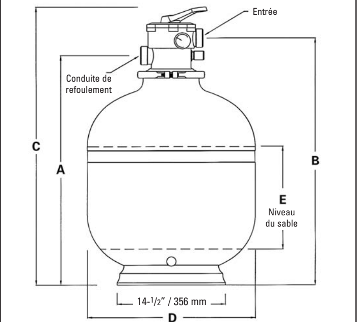
FIGURE 6 - Dimensions pour filtre de sable seulement
