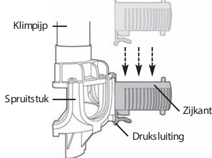
AFBEELDING 1 drukvast detail.
