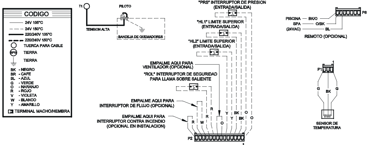
Fig. 21: Diagrama Electronico - Modelo 156 (Calentadores Fabricados Para Chile)
